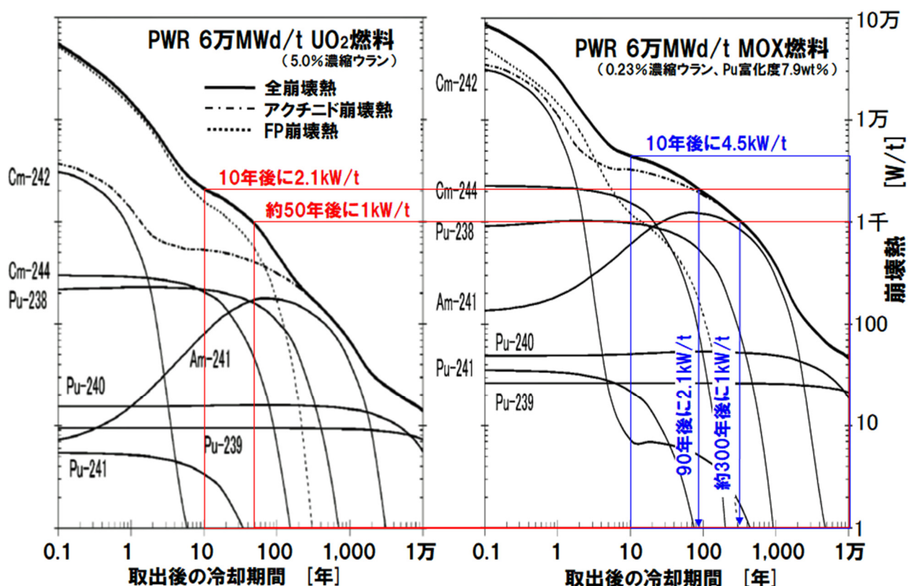
図2. PWR 使用済ウラン燃料(左)と軽水炉使用済 MOX 燃料(右)の原子炉取出後の経過年数(プール冷却期間)と崩壊熱の推移 (注1) (燃焼度は 6 万 MWd/tUO 2 燃料(5.0%濃縮ウラン)と 6 万 MWd/tMOX 燃料(0.23%濃縮ウラン、Pu 富化度 7.9wt%) ;使用済ウラン燃料の崩壊熱は、運転停止直後 2,200kW/t、1 ヶ月後 55kW/t、5 年後 3kW/t、10 年後 2.1kW/t、50 年後 0.94kW/t、100 年後 0.5kW/t と推移する)
