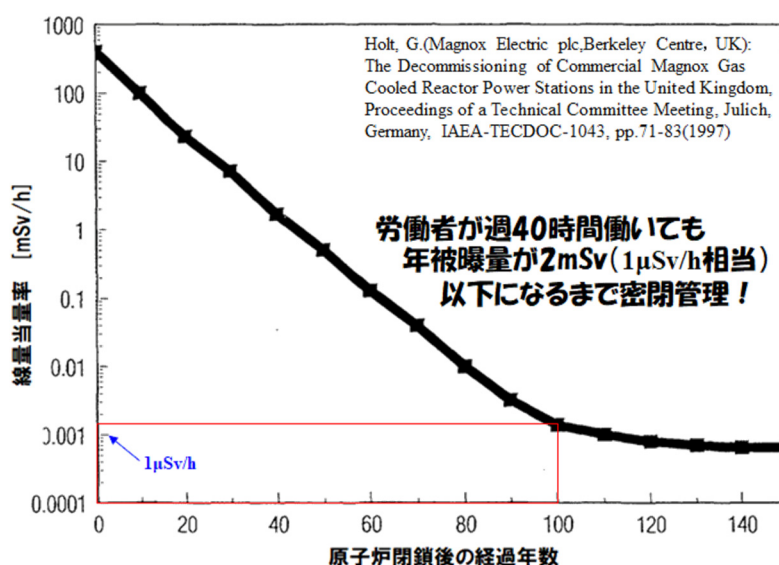
図 1. 英マグノックス代表炉の内部における線量当量率の原子炉閉鎖後の経過年数に伴う減衰状況
