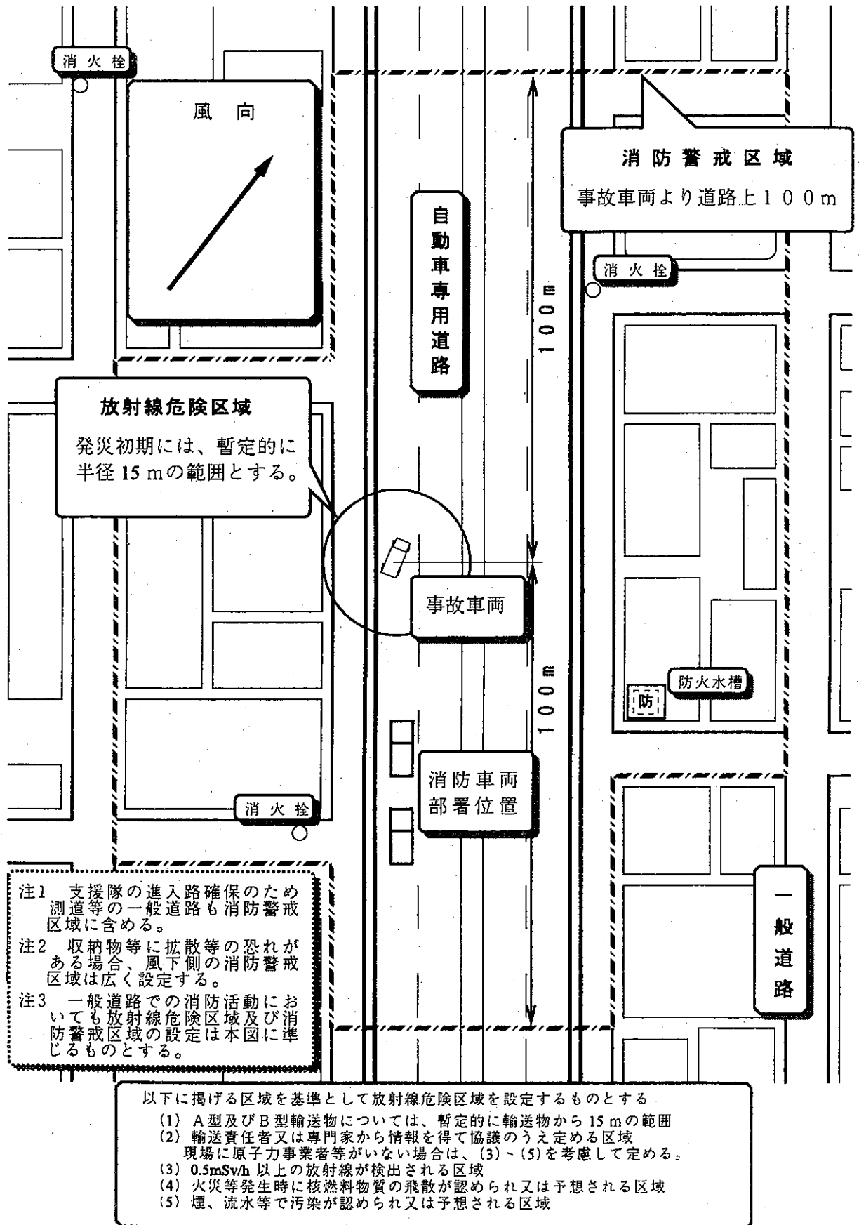
図4-1 計画指針（自動車専用道路の場合）の表示図例
